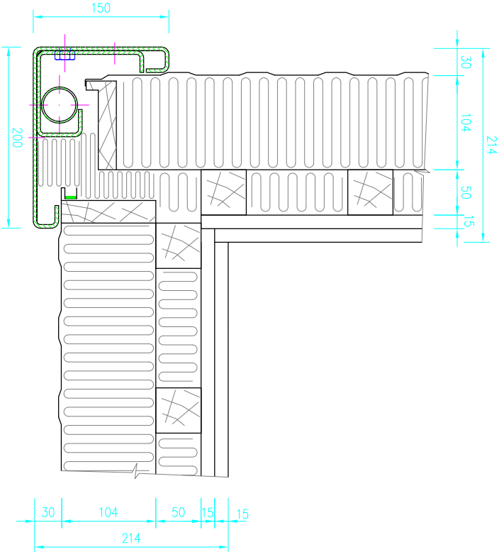
WAND - WAND
