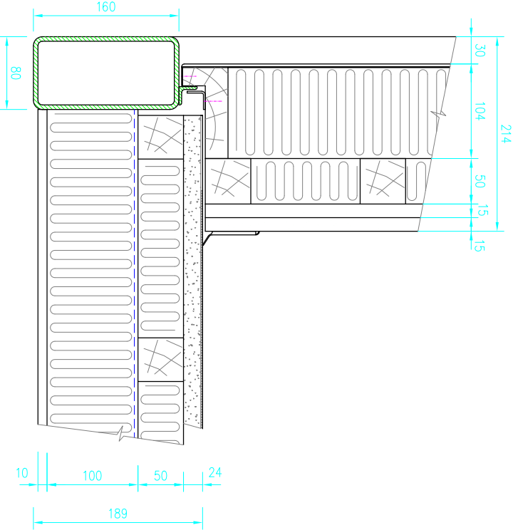
WAND - VLOER
